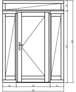
Egyszárnyú + 2 fix oldalvilágító + fix felülvilágító
