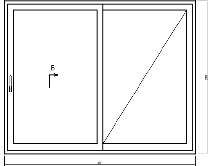
"D" séma 2 emelő-toló mozgó szárny
